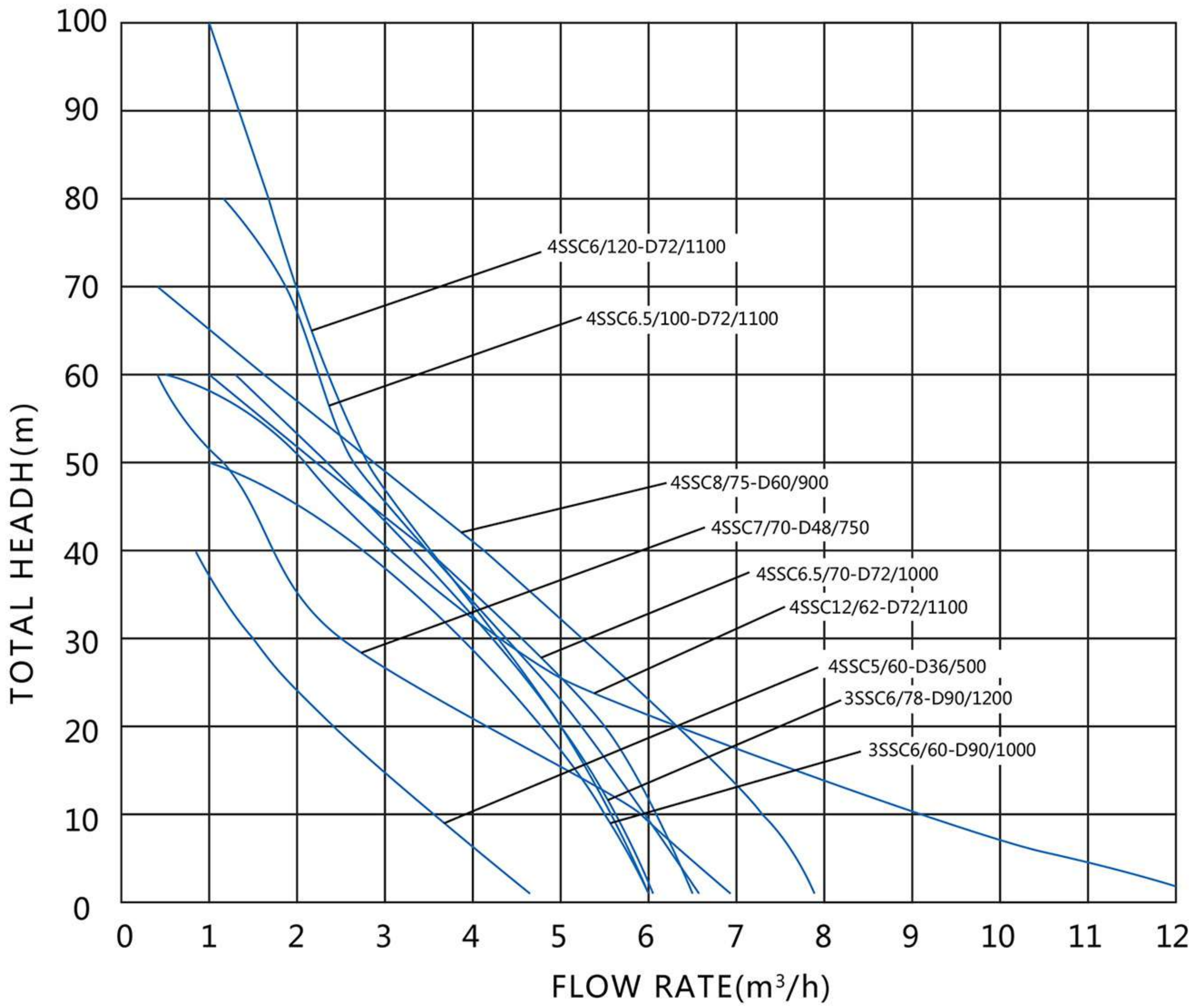
Performance Chart 流量扬程参数
